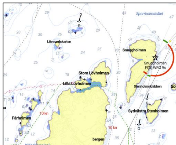
Utdrag från sjökort från applikationen från Skippro. På bilden kan man se att det framgår en fartbegränsning på 10 knop i farleden vid Vaggön.
